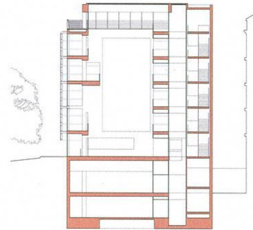
SECCION TRANSVERSAL 03. ESCALA 1/350.
