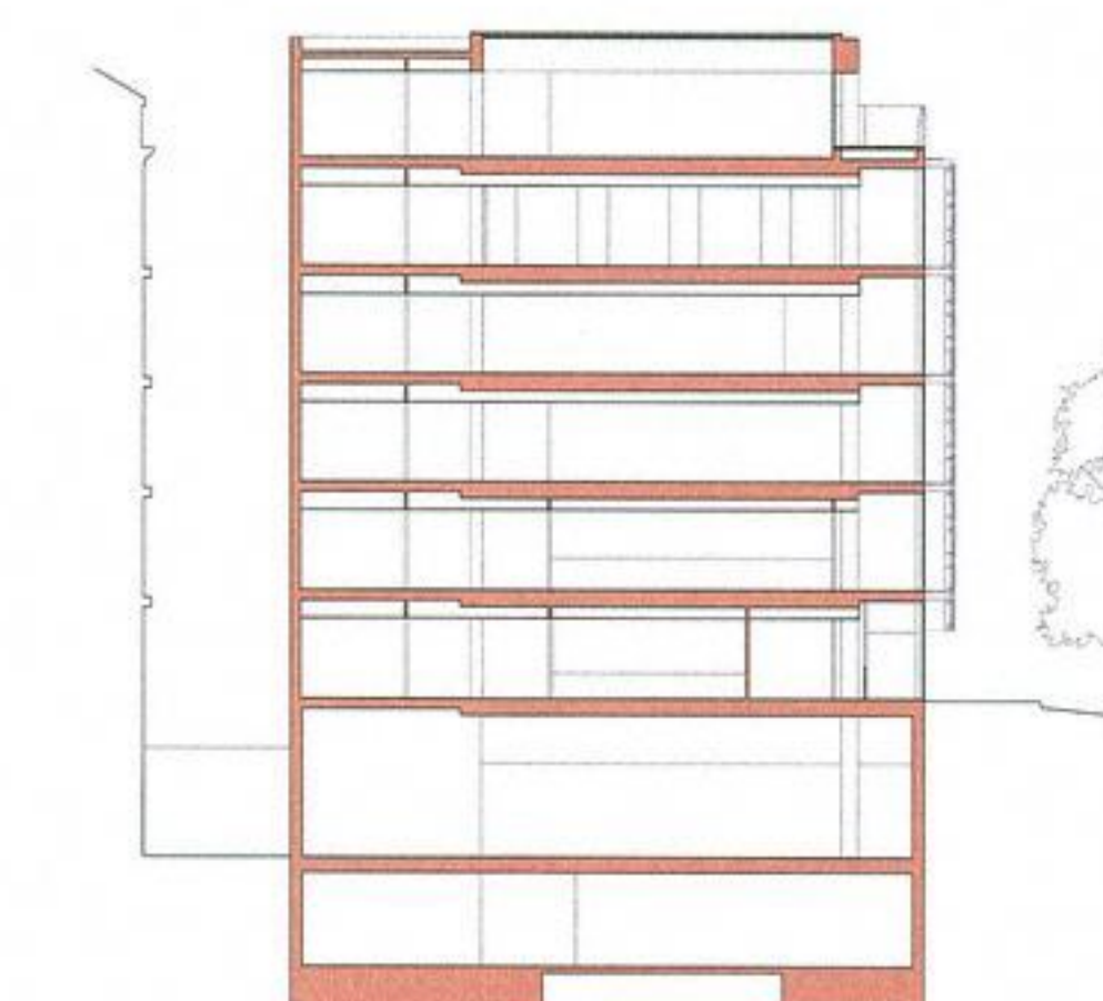
SECCION TRANSVERSAL 04. ESCALA 1/350.
