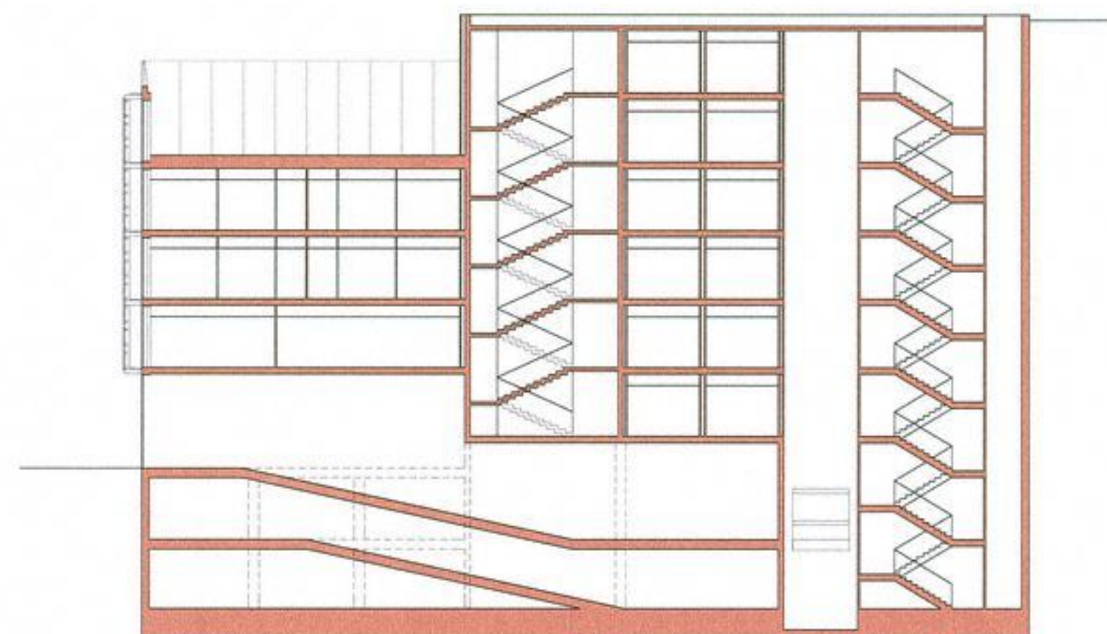
SECCION LONGITUDINAL 01. ESCALA 1/350.
