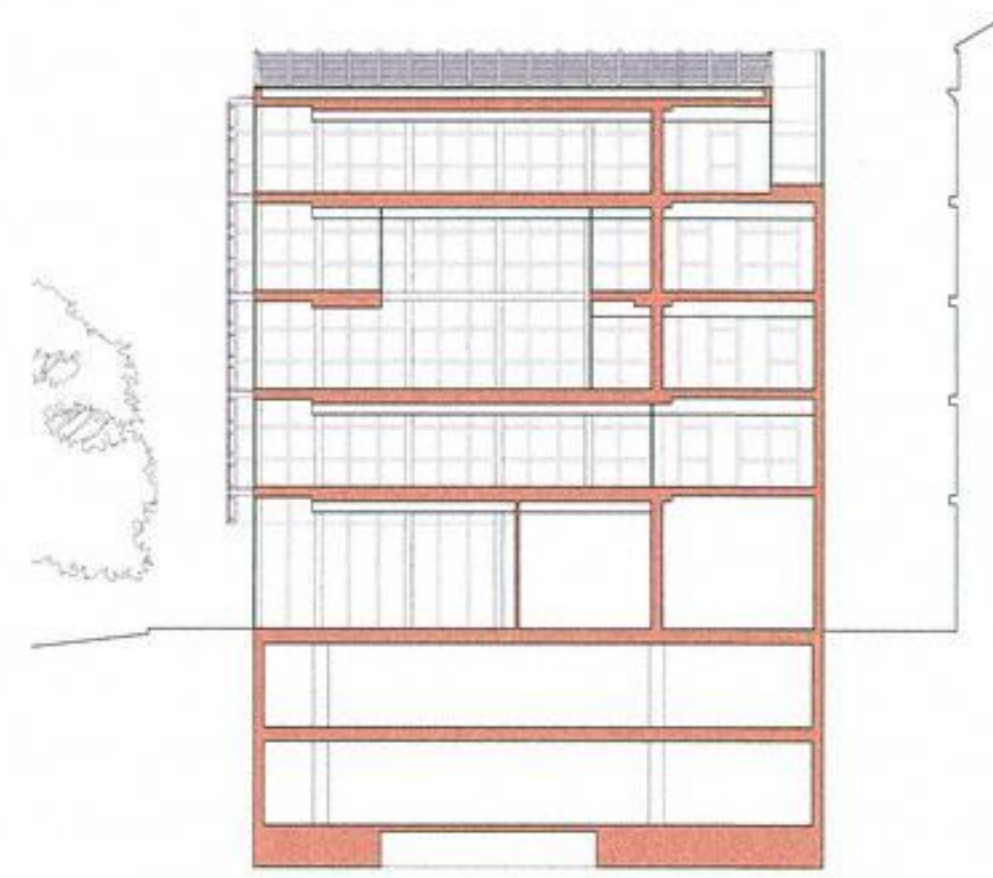
SECCION TRANSVERSAL 01. ESCALA 1/350.
