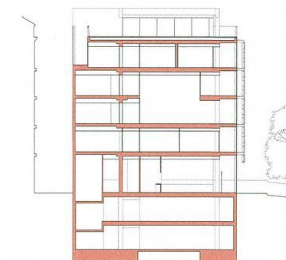
SECCION TRANSVERSAL 02. ESCALA 1/350.
