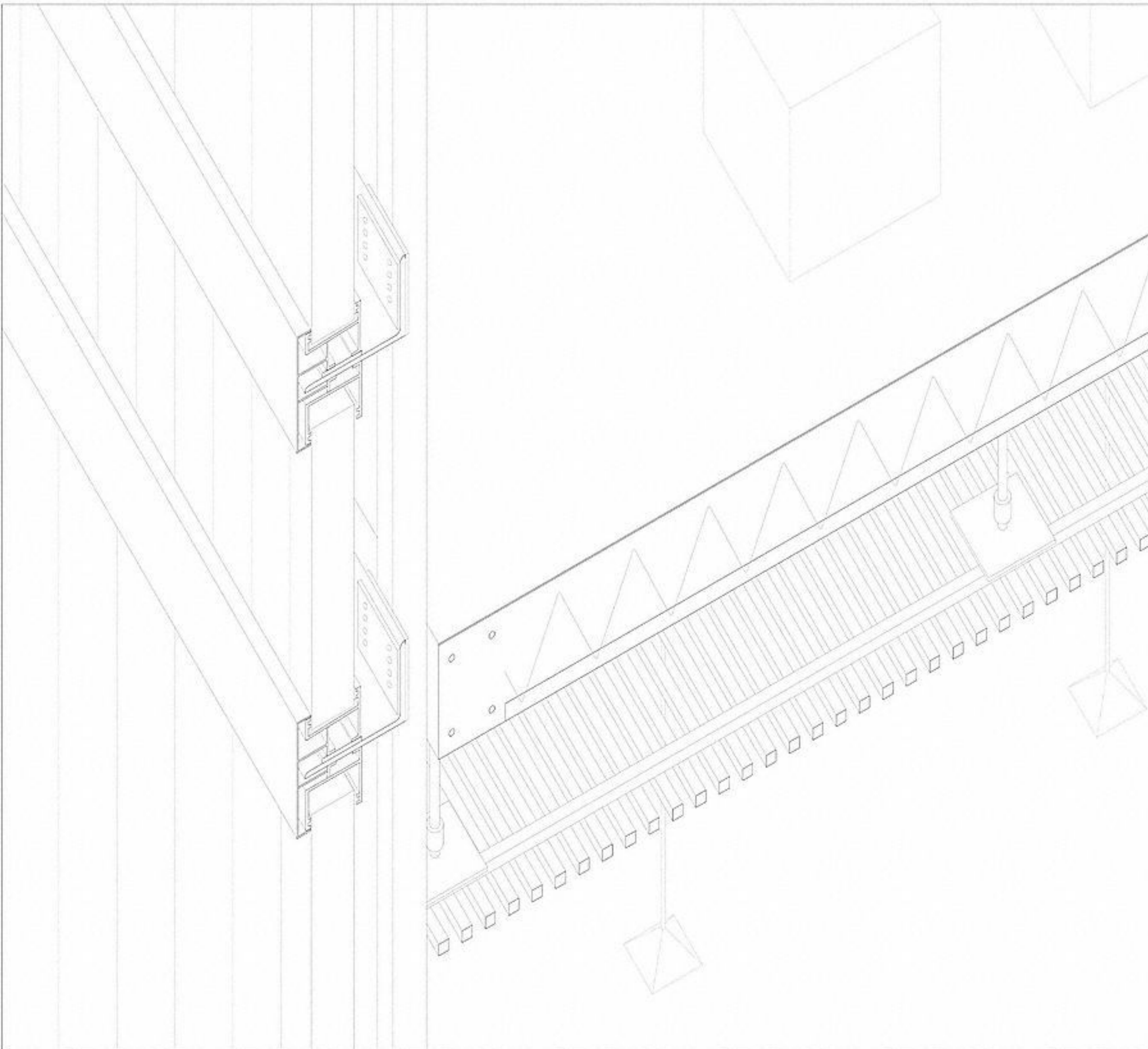
Forjado existente . cerramiento 1 sustitución del existente . 1 : 10
