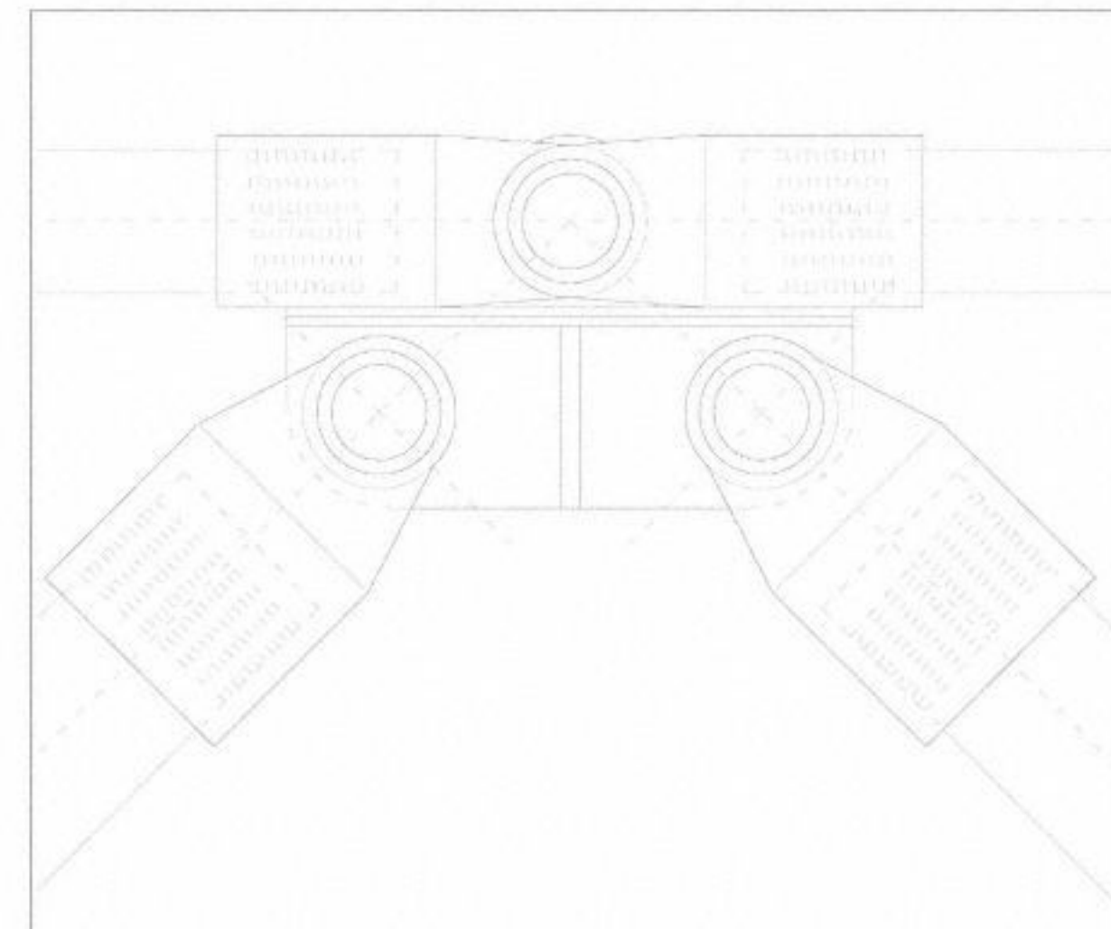
.Detalle nudo superior . 1 : 2
