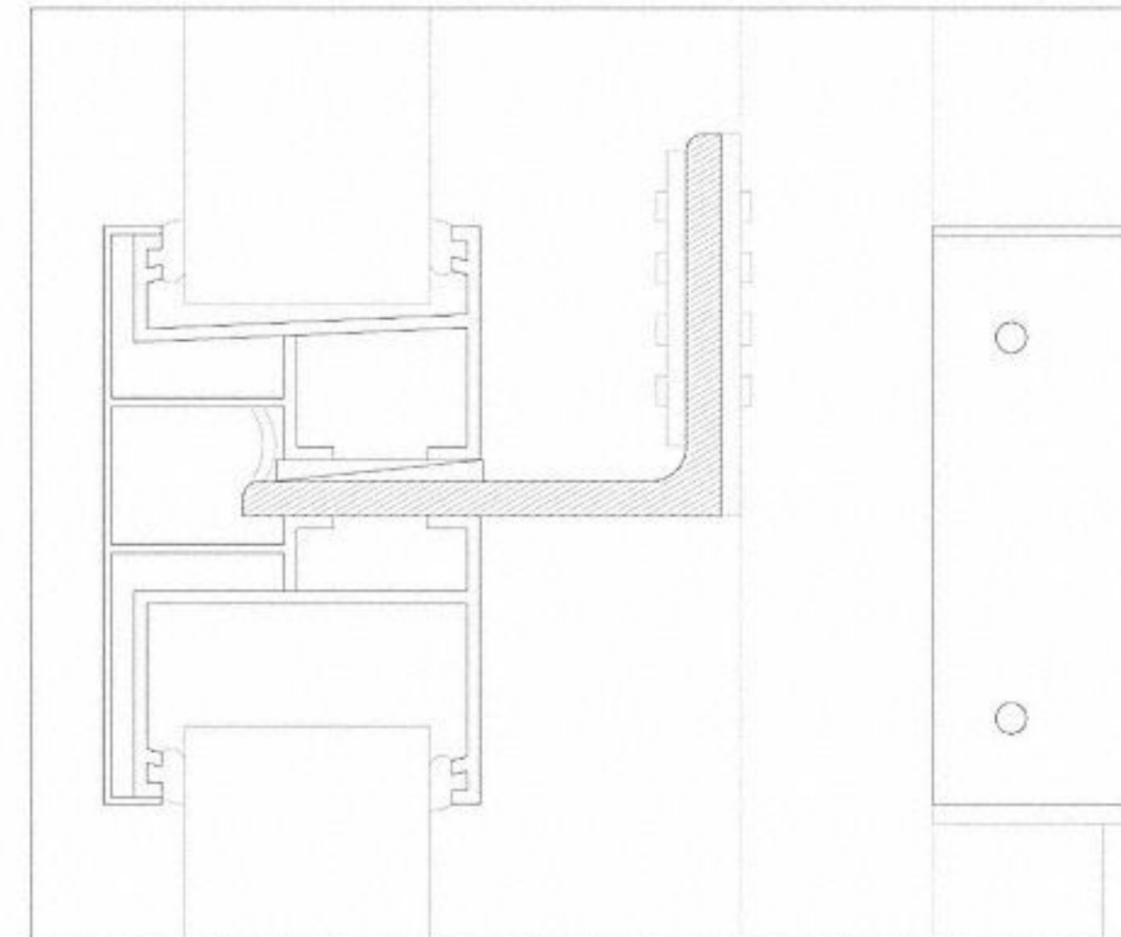
.Cerramiento 1 . detalle . 1 : 5
