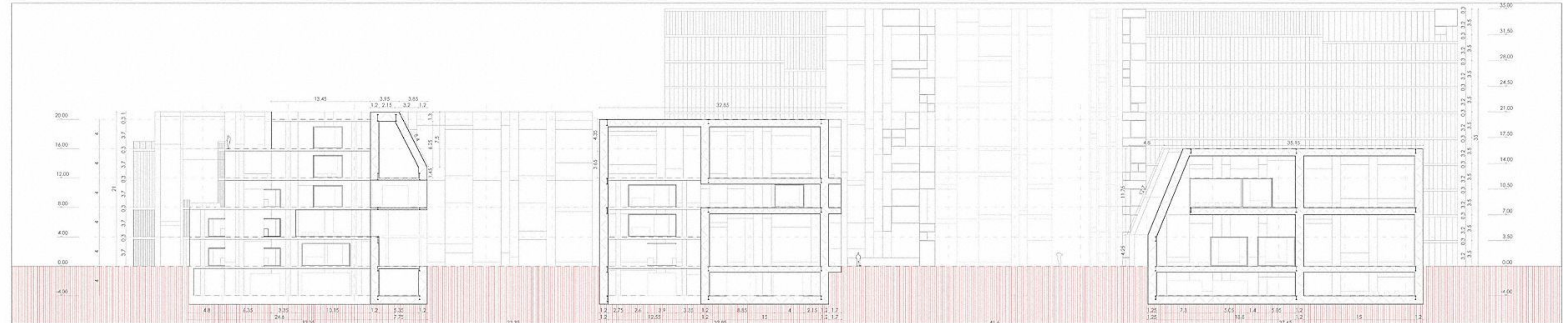
.Manzana B . sección . 1 : 450
