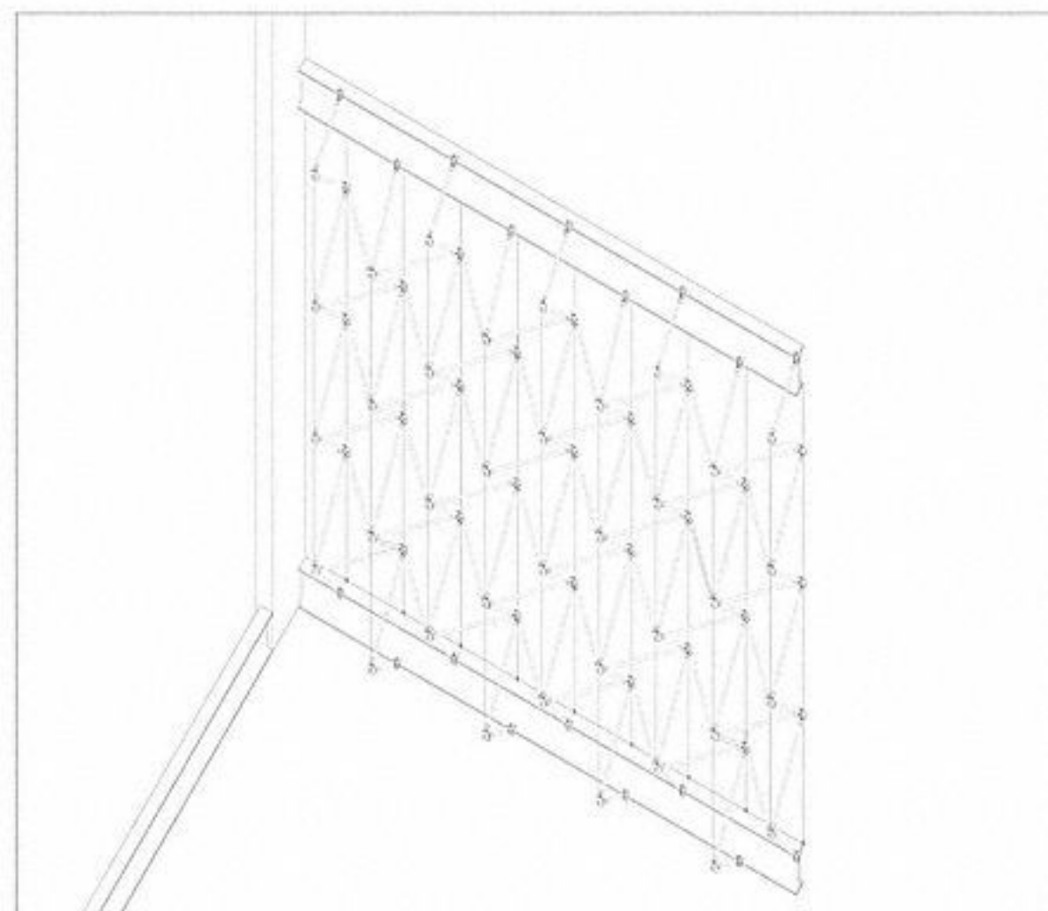
. Cerramiento 2 . estructura secundaria
