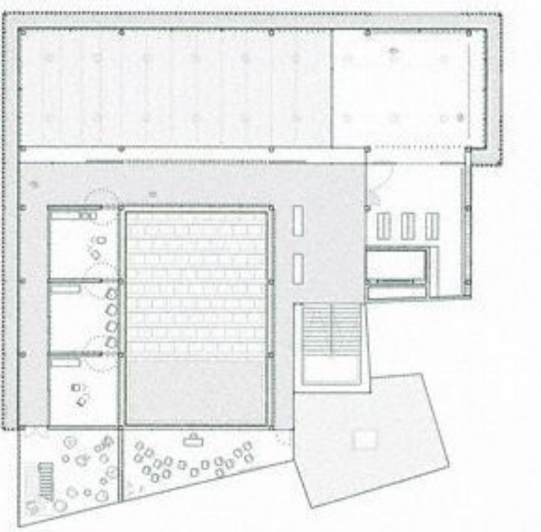
Planta Segunda (+7.80 m) E: 1/500
