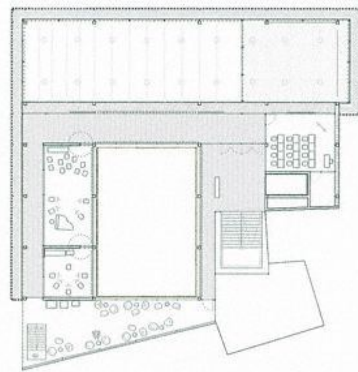
Planta Tercera (+11.15 m) E: 1/500
