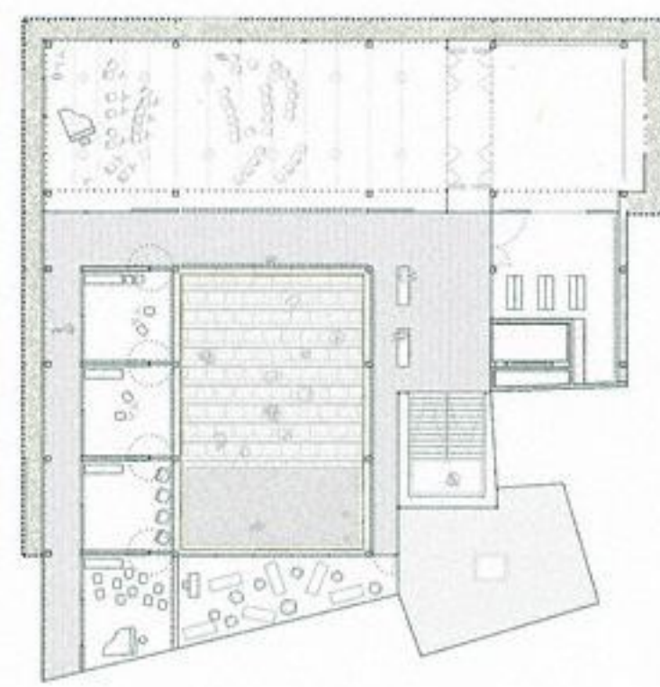
Planta Primera (+4.05 m) E: 1/500
