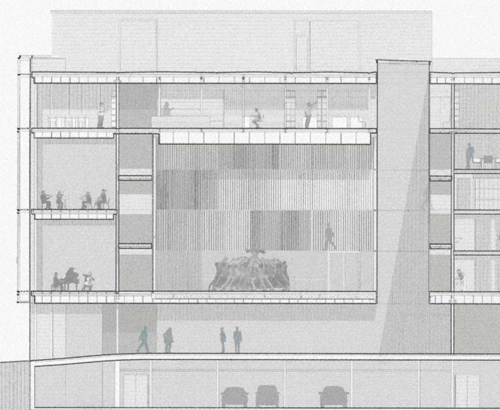
SECCIÓN B-B' E: 1/200
