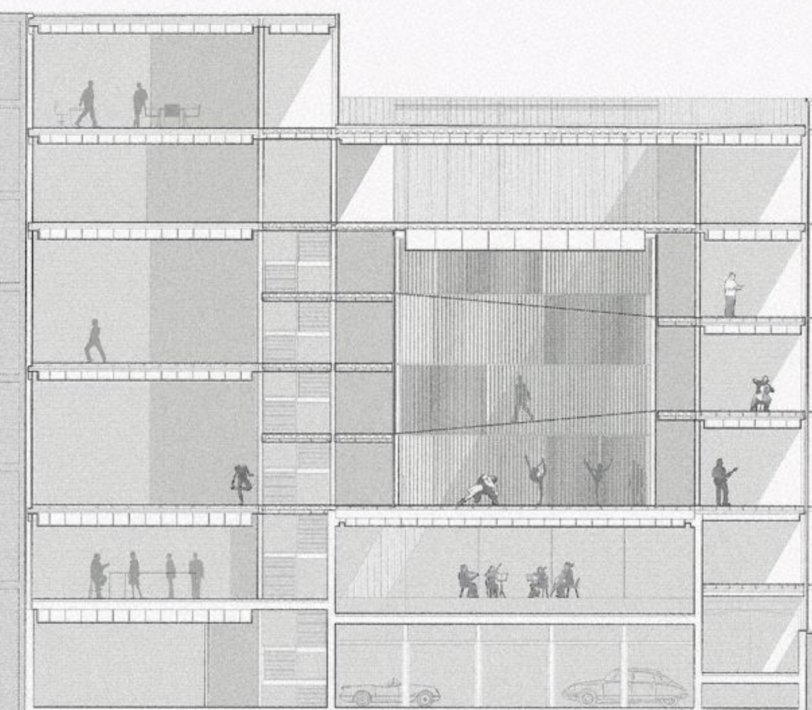
SECCIÓN A-A' E: 1/200
